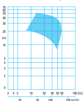
CMX 13... -2 pole
