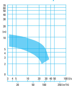
CMX 13... -4 pole
