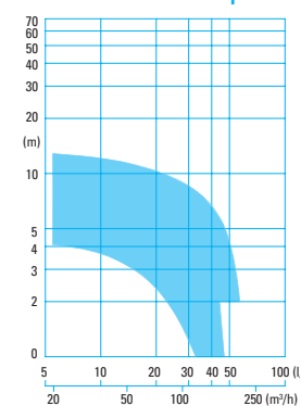
CMX 24... -6 pole
