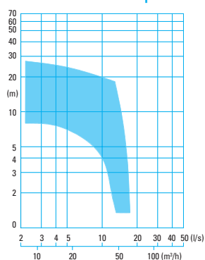
CTP... -2 + 4 pole
