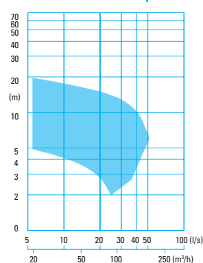
CMX 23... -4 pole
