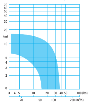
CV(X) 13... -4 pole
