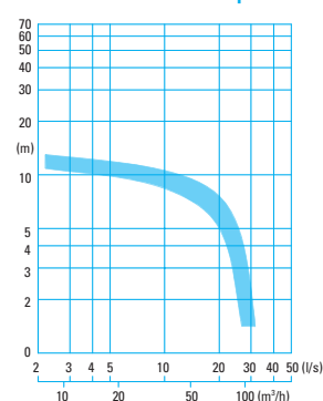
CTP... -4 pole
