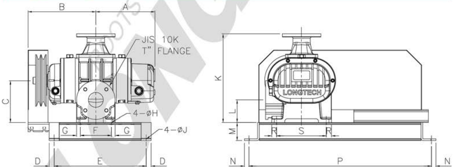
Wt.(Kgs):Main Body Weight Unit:mm
